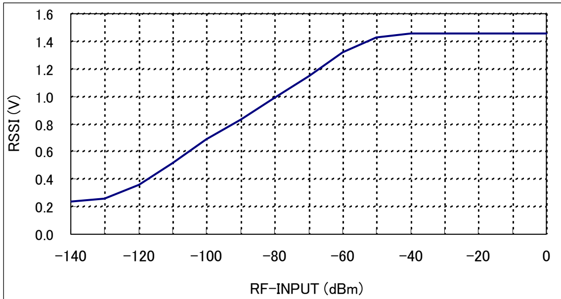
RSSI (V)
